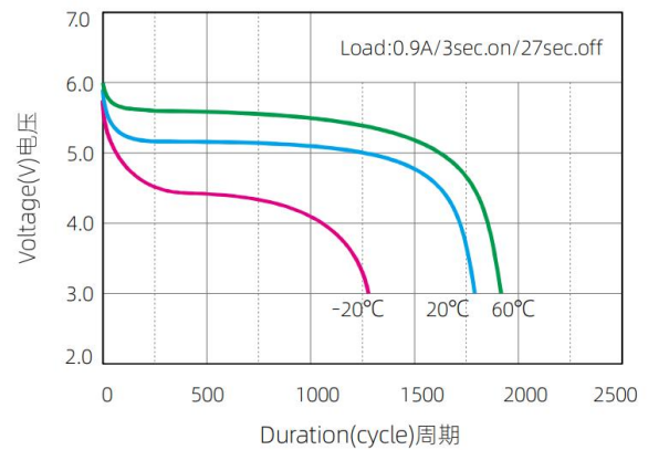
Pulse Discharge 脉冲放电
