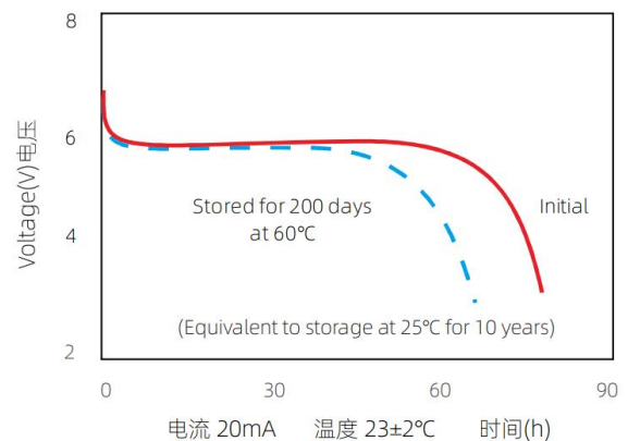
Storage characteristics 存储特性
