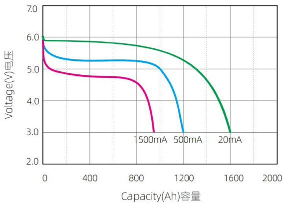
Discharge characteristic 放电特性 (25°C)
