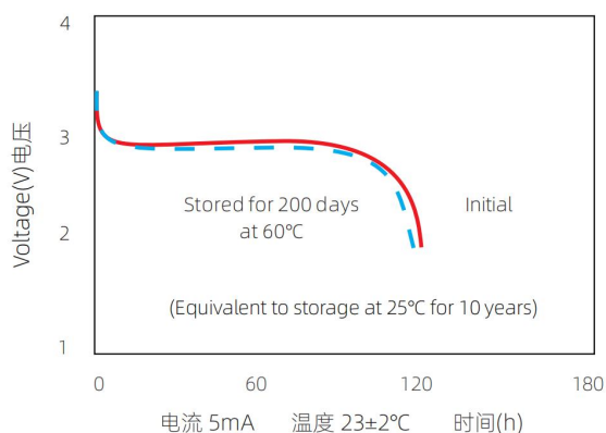
Storage characteristics 存储特性
