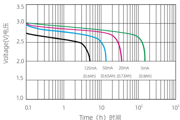
Discharge characteristic 放电特性 (25°C)
